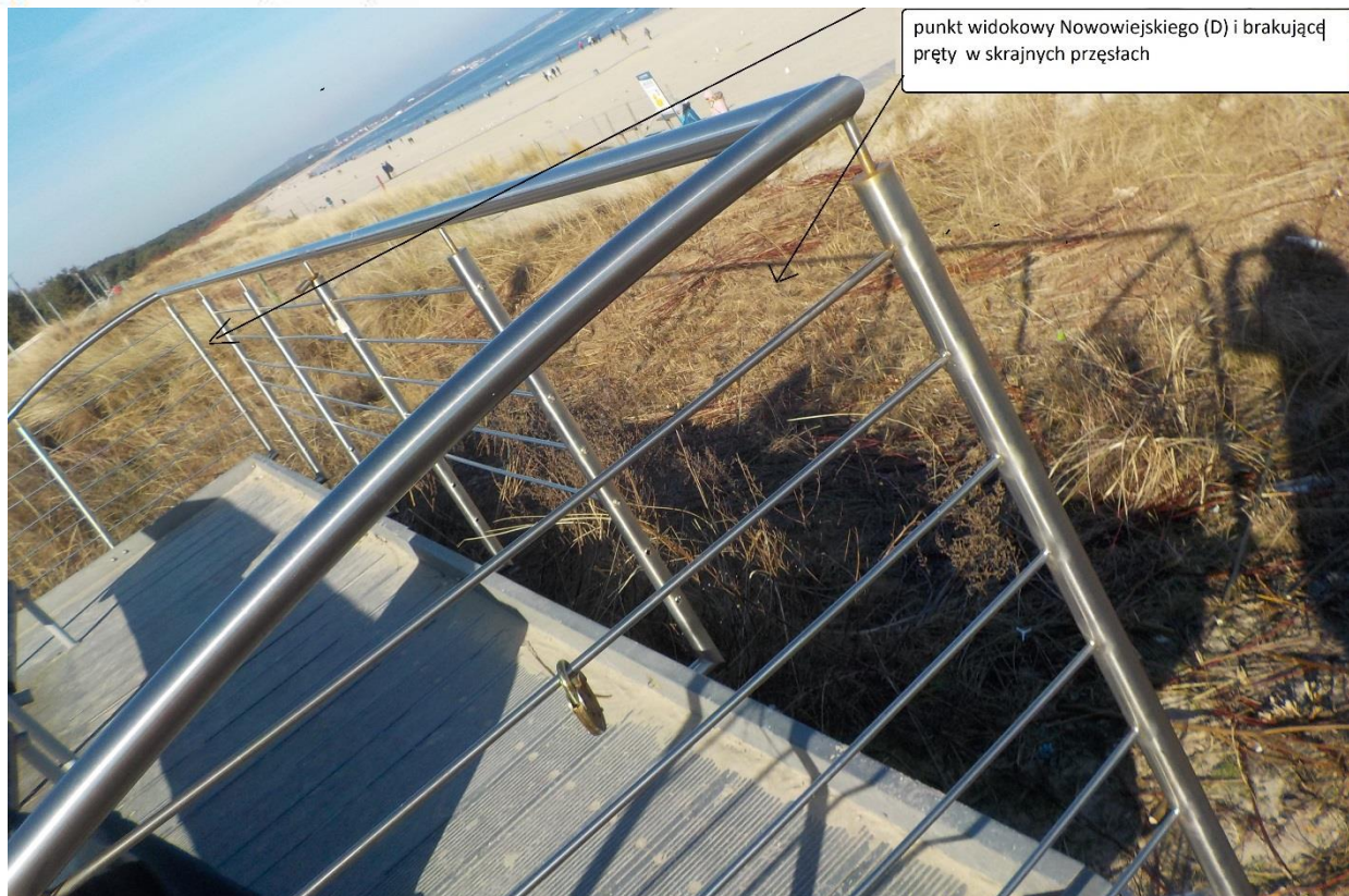
Wejście D od ul. Nowowiejskiego - prawa strona wjazdu dla niepełnosprawnych - częściowe ubytki prętów w przęsłach - wymóg uzupełnienie braków
